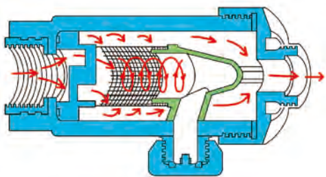
YAMAHO漩渦式過濾管S型水流方向
