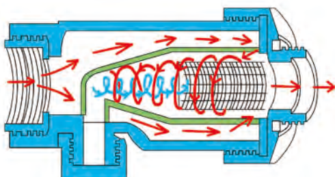
YAMAHO螺旋式過濾管水流方向
