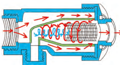
YAMAHO螺旋式過濾管水流方向
